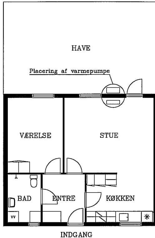
TYPE 01 KASTANIE ALLE 1A-1H & 3A-3L
